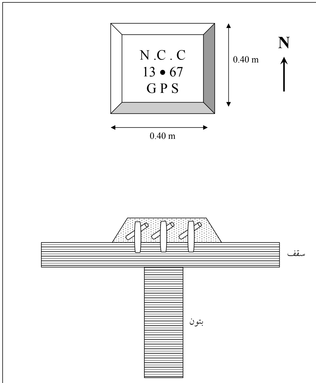
شکل ۶ - مقطع ایستگاههای اصلی GPS روی پشت بام
