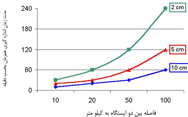
نمودار ۲-۱ رابطه بین زمان اندازه گیری، طول باز و دقت قابل حصول به نقل از سایت National GPS Network
