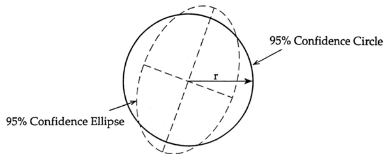
بیضی خطا و دایره اطمینان ۹۵٪
